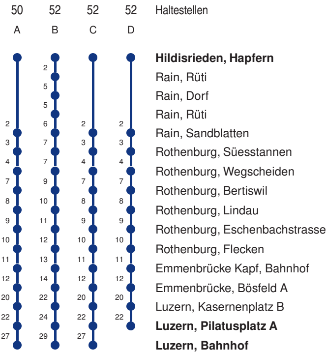
Linienvverläufe mit ca. Reisezeit in Minuten
